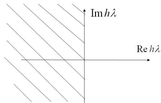
Рис. 1. Область абсолютной устойчивости (заштрихована) AL-устойчивых методов интегрирования
