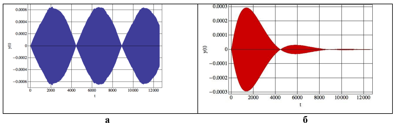
Рис. 2. Решение задачи ТЕСТ 4 при TOL = 0.001, а - метод BDF из библиотеки C-Library NAG, б - метод M3 из Си библиотеки SADEL.
